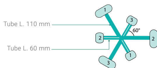
Montage des 6 patères (niveau 1 en bas)
