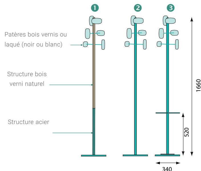
Portemanteaux Épi 6 patères
