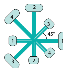
Montage des 8 patères (niveau 1 en bas)
