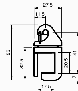
Schéma du profil moteur à droite
